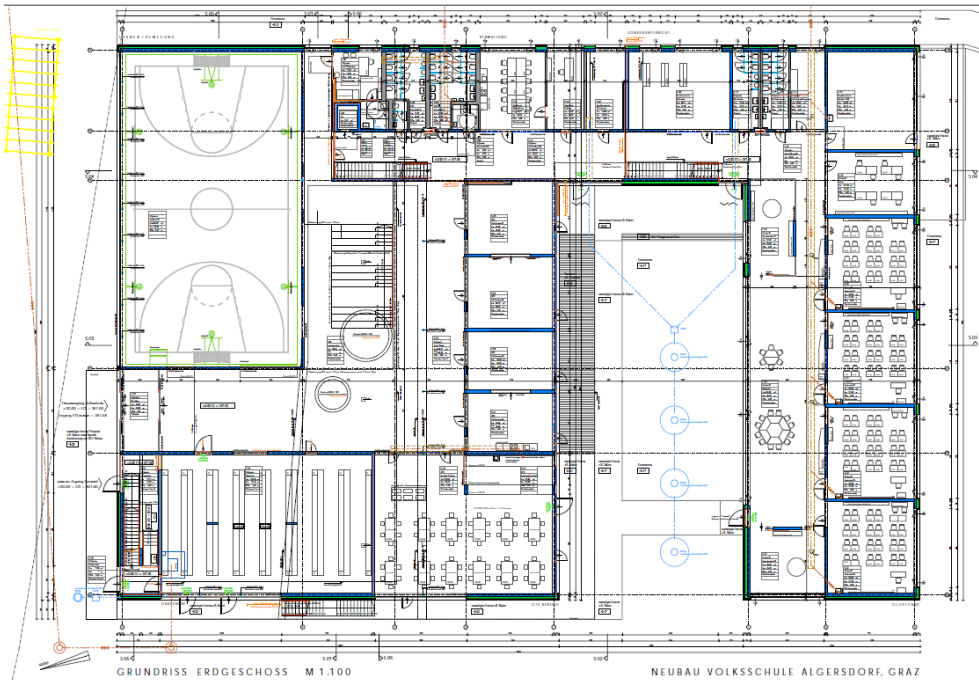
Abbildung 4: Einreichplan VS Algersdorf EG Quelle: GBG - Einreichplan
