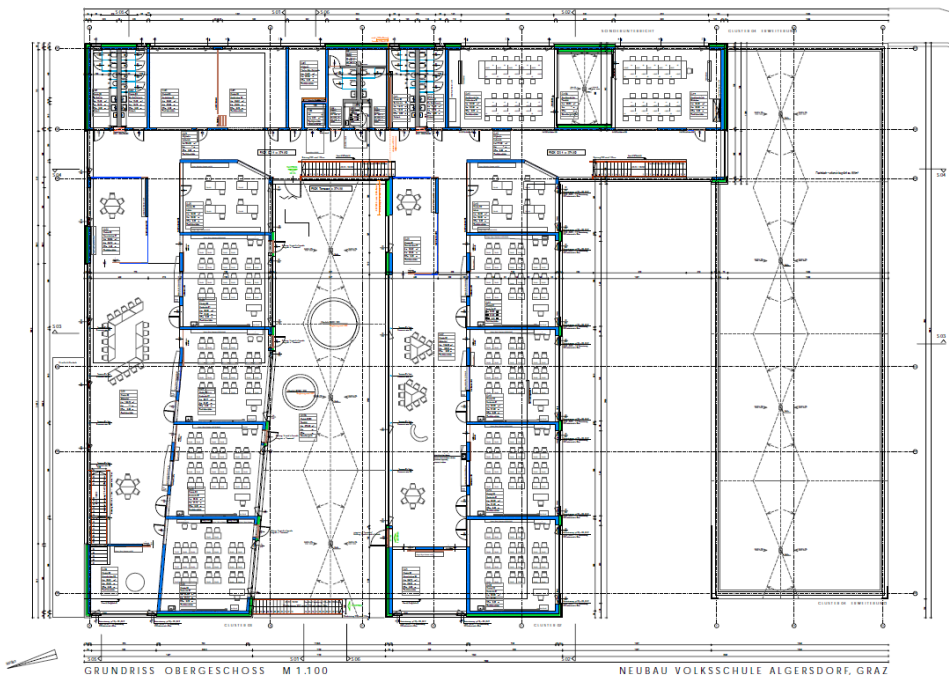
Abbildung 5: Einreichplan VS Algersdorf OG Quelle: GBG - Einreichplan
